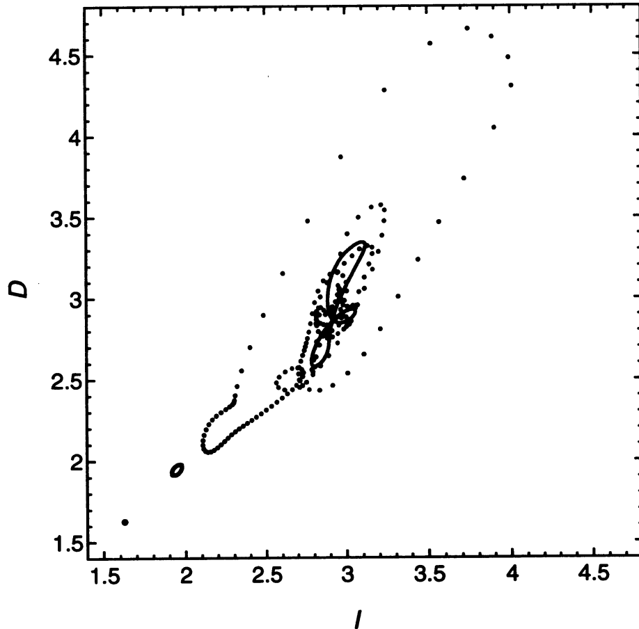
図 5. パースト軌道と 2 つの周期軌道の (I, D) 面への射影. 時間 400h/U にわたるパースト軌道を細い灰色の線で示す. この軌道には 2h/U ごとに黒点が付してある. 閉じた太い黒色の線と太い灰色の線は, それぞれ周期軌道を表す. 黒丸は, 長い流れ方向周期 L_x = 6.189h での Nagata (1990) の (下分枝) 定常解を示す. この定常解は太い黒色の周期軌道に分岐する. 太い灰色の周期軌道は図 1, 2 の周期軌道と同一である.
