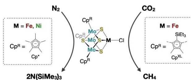
Figure 1. 立方体型 [\text{Mo}_3\text{S}_4\text{M}] クラスターの構造とその \text{N}_2 ならびに \text{CO}_2 還元反応.
