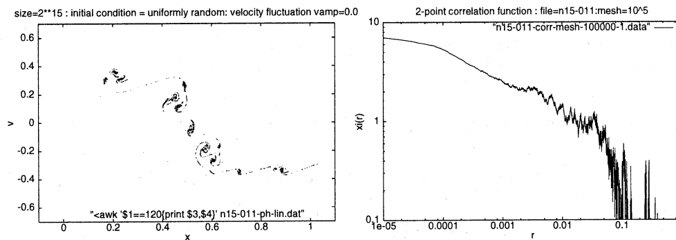
Figure 1: (左図)：初期条件が v_i(0) = 0 , x_i(0) = 区間 [0, 1] の一様乱数の場合の (x_i, v_i) の分布。 N = 2^{15} , t = 9.375 。 (右図)：このときの2点相関関数 \xi(r) 。べき相関 \xi(r) \propto r^{-\alpha} が見られる。
