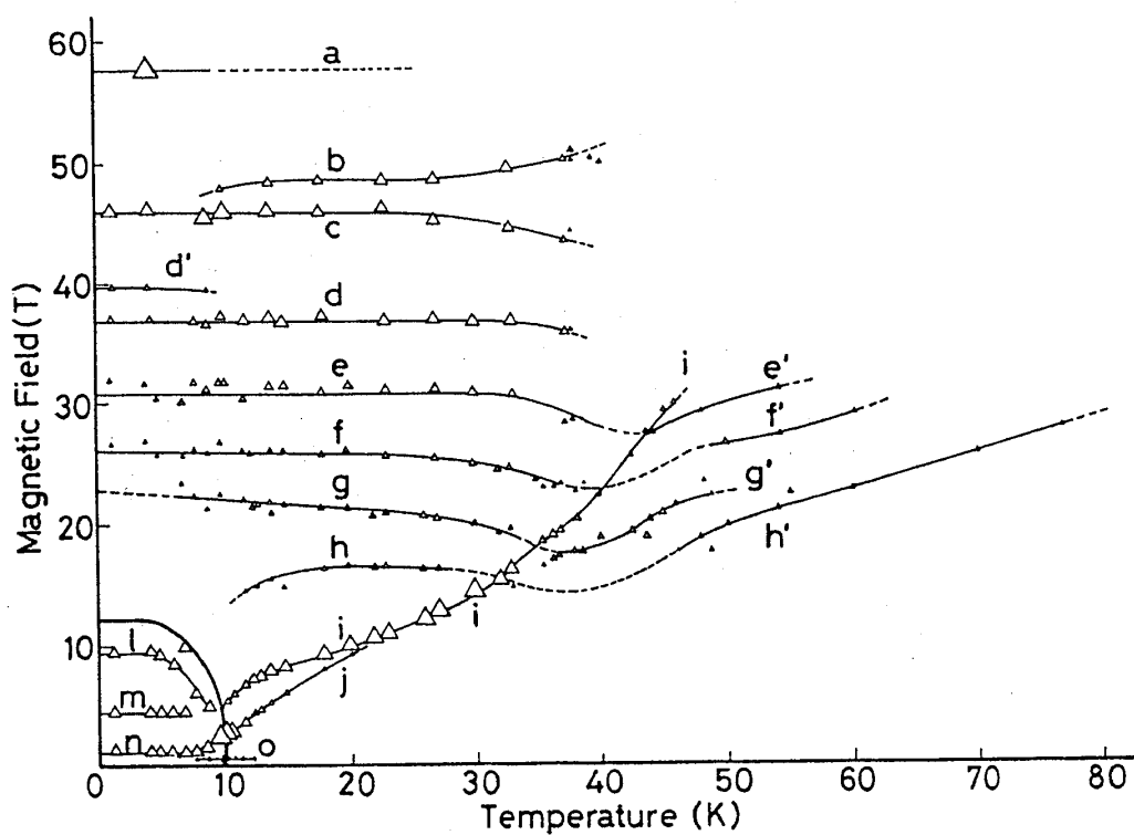
図11 強磁場磁気相図（上り磁場）。a～nは図8に対応した、磁化のとびを示す。 \Delta の大きさは微分帯磁率のピークの高さを示している。太線は \Gamma の反強磁性の境界を示す。磁場を[100]方向にかけている。
