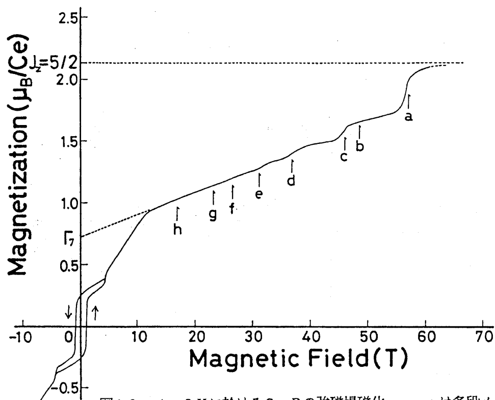
図10 4. 2 Kに於けるCePの強磁場磁化。a～gは多段メタ磁性の磁化の飛びを示す。
