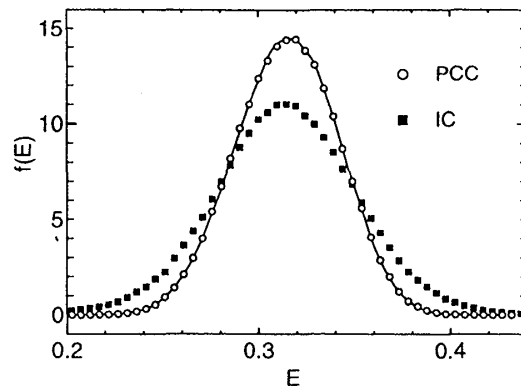
図 2: PCC アルゴリズムと IC アルゴリズムによるエネルギーヒストグラム f(E) . 2次元イジングモデルでサイズは L = 64 で topological 規則の結果. 温度一定の計算によるエネルギーヒストグラムを実線により示してある.
