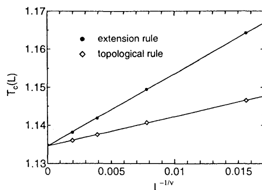
図 1: 2次元イジングモデル ( q = 2 ) の T_c(L) のサイズ依存性. L^{-1/\nu} の関数としてプロット. 但し, \nu=1 . また系のサイズは L = 64, 128, 256, 512 .
