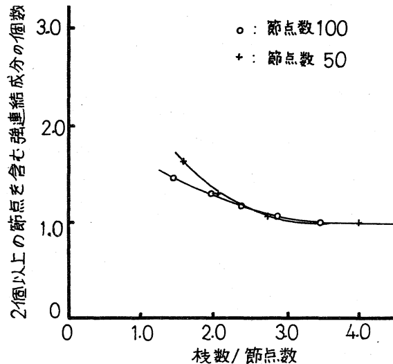
図9. 2個以上の節点を含む強連結成分の個数と枝数/節点数の関係
