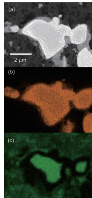
図7 半放電した活物質のSEM(a)反射電子像とエネルギー分散型X線分光法で得られた(b)BiMα 1 , (c)F-Kα 12 のマッピング像。粒子の外側がBi, 内側がBiF 3 で構成されており、脱フッ化反応が粒子の外側から進行することを示している (Reprinted with permission from Ref. 25, Copyright 2019 American Chemical Society)。
