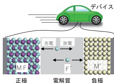
図2 フッ化物イオンシャトル二次電池の稼働原理図。Mは金属元素、M'はMとは異なる金属元素を示している。紫丸は金属イオン、水色丸はフッ化物イオン、黄色丸は紫丸とは異なる金属原子、灰色部分は電解質を示している。電解質中をフッ化物イオンがシャトルしている様子を示している（カラー図はWeb版を参照）。
