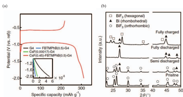
図 4 有機電解液を用いた \text{BiF}_3 電極の脱フッ化、フッ化反応の実証。(a) 定電流充放電曲線。赤線が CsF, FBTMPhB, テトラグライムから調製した電解液を用いた場合に得られた曲線である。(b) XRD による電極の結晶構造解析。下から、Pristine (放電前), Semi discharged (満放電の半分の容量を放電した後), Fully discharged (満放電後), Fully charged (満充電後) の電極から得られた X 線回折パターン。白丸は orthorhombic 相 \text{BiF}_3 、黒三角は rhombohedral 相 Bi、白四角は hexagonal 相 \text{BiF}_3 の結晶構造に起因する回折ピークである。この結果から、放電前は \text{BiF}_3 のみが存在するが、放電後に Bi と変化し、充電後に大部分が \text{BiF}_3 に変化することがわかった (Reprinted from Ref. 14.)。
