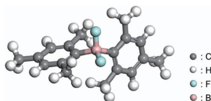
図3 第一原理計算で最適化したフッ化物イオンを配位した fluorobis(2,4,6-trimethylphenyl)borane (FBTmPhB) の分子構造。灰丸は炭素、白丸は水素、水色丸はフッ素、桃色はホウ素を示している（Reprinted from Ref. 14.）（カラー図はWeb版を参照）。
