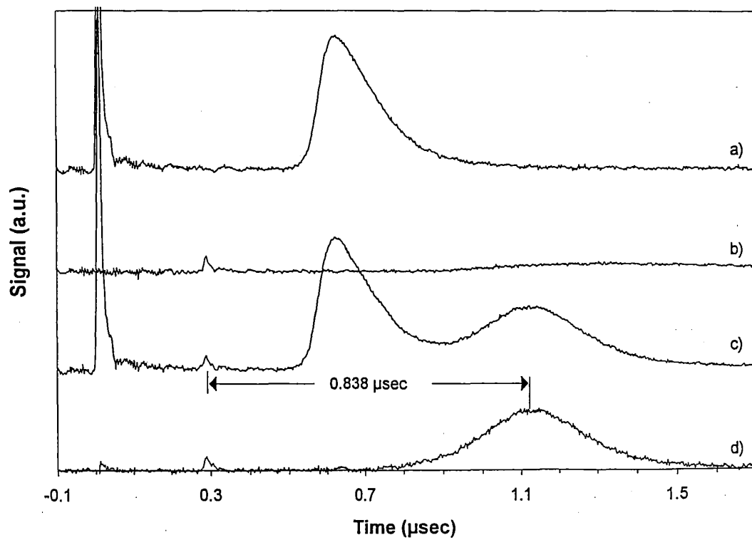
図1. 2連続パルス励起下における励起子パルス伝播を示す実験 2) 。(a)単一パンプパルス励起の場合。(b)単一プローブパルス励起の場合。(c)パンプとプローブパルス励起による信号。(d) (c)と(a)の信号差を示す。
