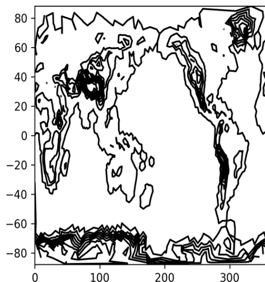
図 2 モデルの地形。
