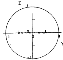
第1図。 3面図による渦糸の時間発展。(a) 2つの渦輪、(b) みつわ形の渦糸、 (c) 球内の渦輪。
