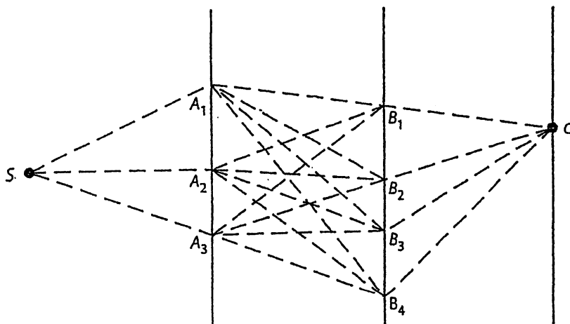
図 6. 2つのスクリーンにいくつかの穴をあける
