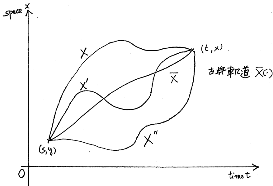
図 1. (s, y) と (t, x) とを結ぶ経路達
