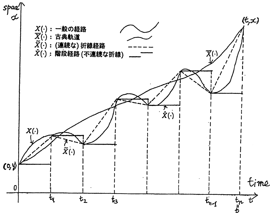
図 2. (0, y) と (t, x) とを結ぶ時間分割近似経路達
