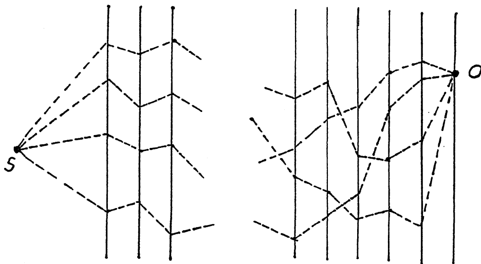
図 7. 沢山のスクリーンに沢山の穴をあける
