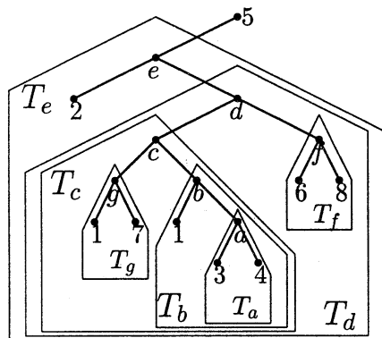
図 2: distortion index の計算 in (T_e, i)
