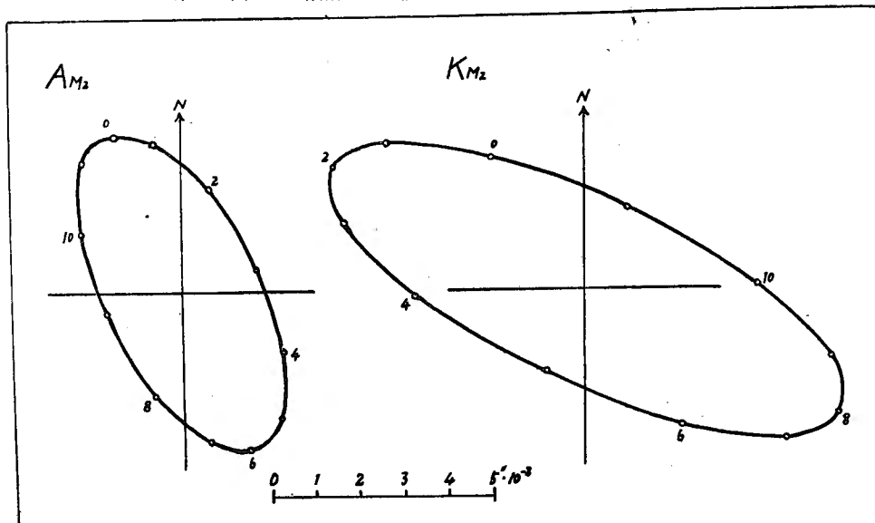
第二圖 地殻潮汐観測値, 阿蘇(A)並上賀茂(K) M_2, O_1
