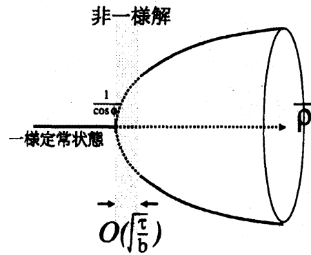
図6: 解の振舞い
