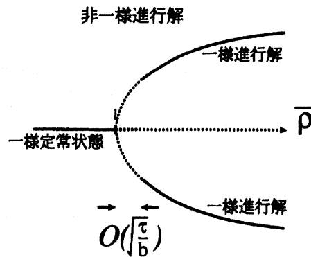
図 2: 解の振舞い
