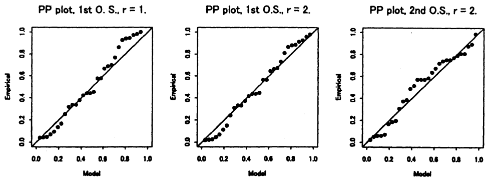
図 8. GEV モデルの下での PP plot, r=1 . 図 9. GEV モデルの下での PP plot, r=2 .
