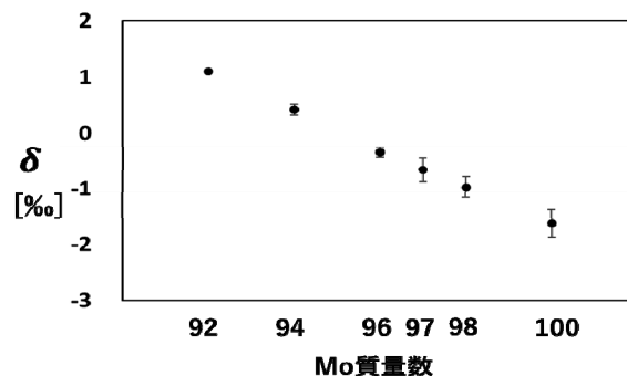
図1 δ 100 Mo 質量数と同位体濃縮係数の関係
