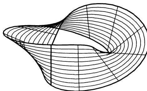
図 3 曲面描画
