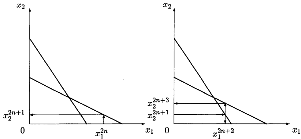
図 2. 最適商品生産量の時間的推移
