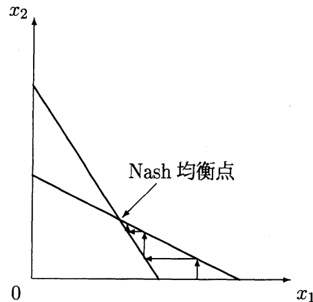
図 3. Nash 均衡点への変移グラフ
