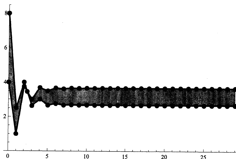
図5. A 社、B 社の生産量
