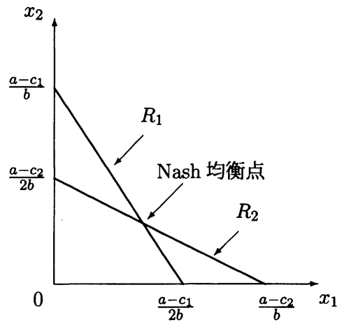
図 1. 各社の反応集合のグラフ
