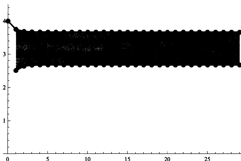
図 4. A 社、B 社の生産量
