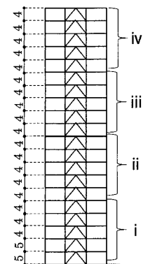
図3 解析モデル
