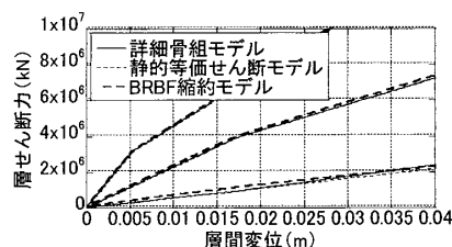
図4 復元力特性
