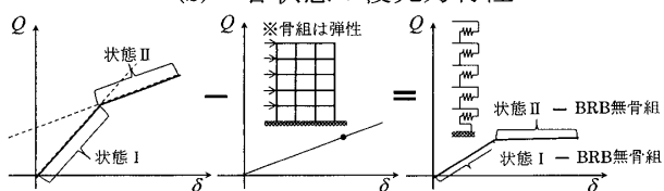
(c) セン断バネの復元力特性決定の手順
