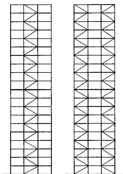
図6 千鳥配置
