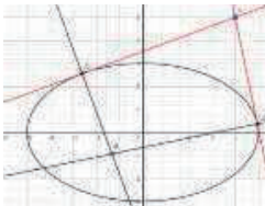
図2. 楕円法線の交点
