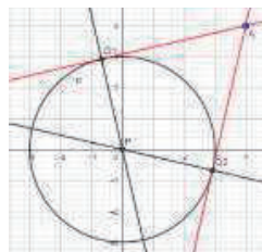
図1. 円での法線の交点
