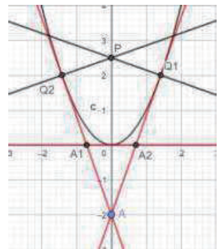
図5. 点Pの原像3点
