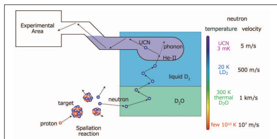
図1 超冷中性子源の原理。陽子ビームによる核破砕反応で発生した高速中性子は、重水および液体重水素減速材によって減速され、超流動ヘリウム(He-II)中での非弾性散乱によって超冷中性子(UCN)に変換される。
