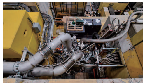
図2 TRIUMFビームライン上に設置されたUCN源
