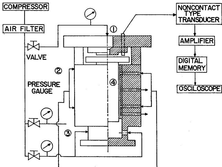
Fig. 25. Experimental apparatus.
