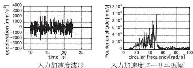
図21 入力特性
