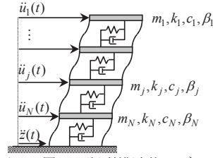
図 1 N 層せん断型構造物モデル
