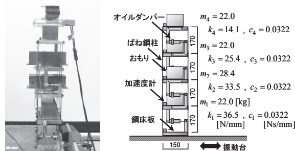
図20 4層せん断型構造物模型
