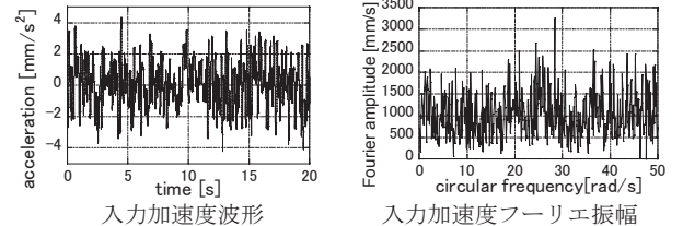
図 5 入力特性
