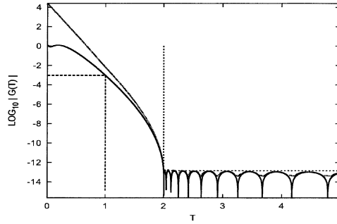
図 10: 最小 2 乗の方法による伝達関数 (その 1): |g(t)| ( n=30, \mu=2.0, \sigma=3.0, \epsilon=10^{-13} ) g_p = 9.2 \times 10^{-4} , g_s = 1.4 \times 10^{-13}
