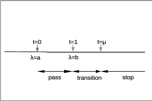
図 1: 固有値 \lambda の区間 [a, b] と正規化座標 t の関係 通過域 \lambda \in [a, b] , t \in [0, 1] ; 遷移域 t \in (1, \mu) ; 阻止域 [mu, \inf)
