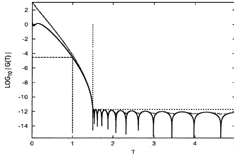
図 11: 最小 2 乗の方法による伝達関数 (その 2): |g(t)| ( n=30, \mu=1.5, \sigma=3.0, \epsilon=10^{-12} ) g_p = 2.9 \times 10^{-5} , g_s = 1.9 \times 10^{-12}
