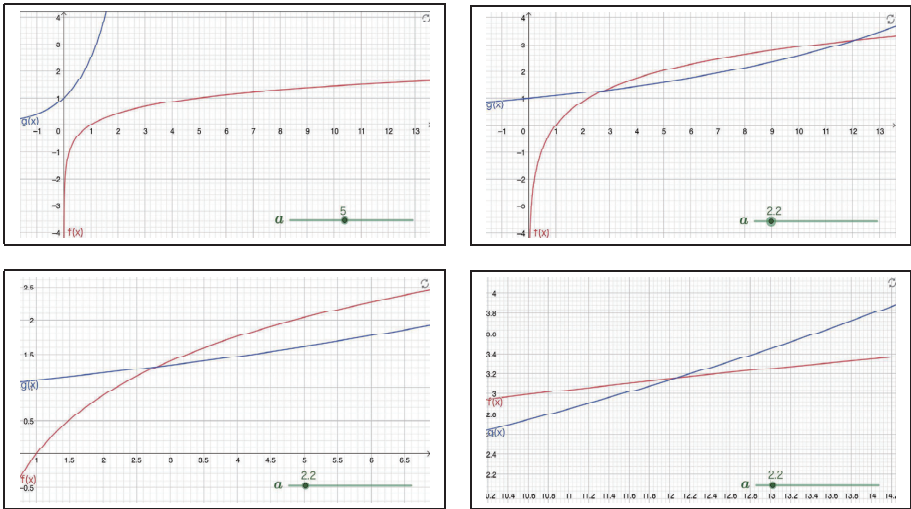
図 2: 対数関数と指数関数のグラフ
