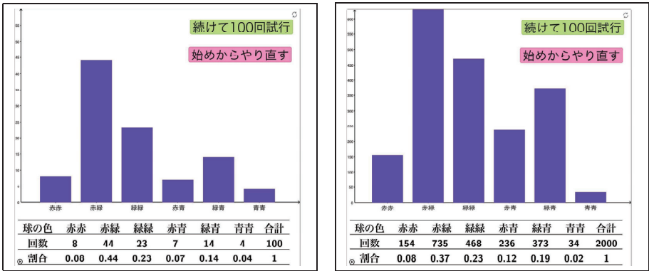
図 3: 玉の取り出し
