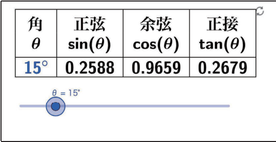
図 1: 三角関数の表
