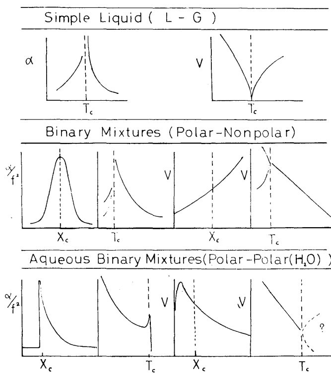
第1図 単純液体、二成分液体の超音波吸収と音速度のタイプと分類
