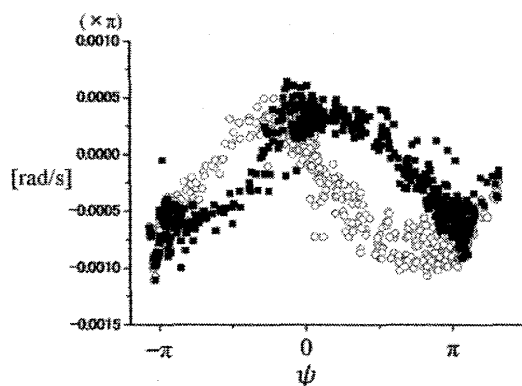
図1. 結合関数 q(\psi) (■)および q(-\psi) - \Delta\omega/\varepsilon (○)。面積比が0.135, 0.066, 0.060, 0.048, 0.031で得られた結合関数の重ね合わせ。
