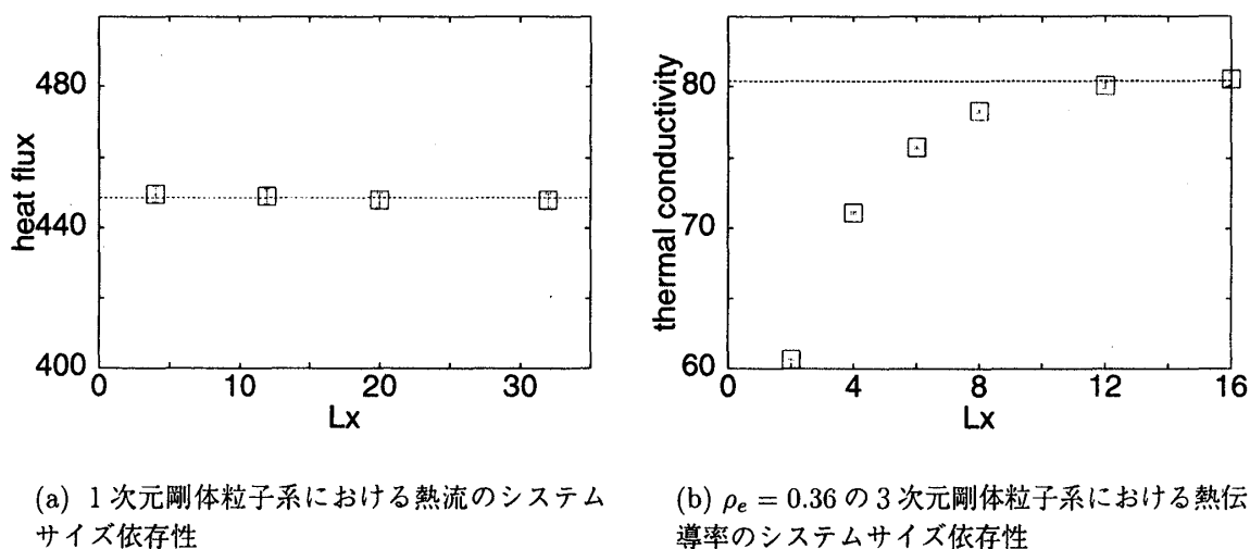
図 4.6: 1次元と3次元でのサイズ依存性
