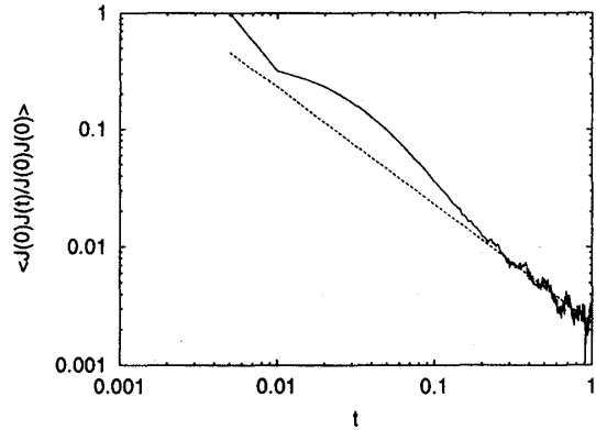
図 5.3: 2 次元の孤立系の熱流の自己相関関数。両対数プロットで示した。直線は \sim t^{-1} の直線。
