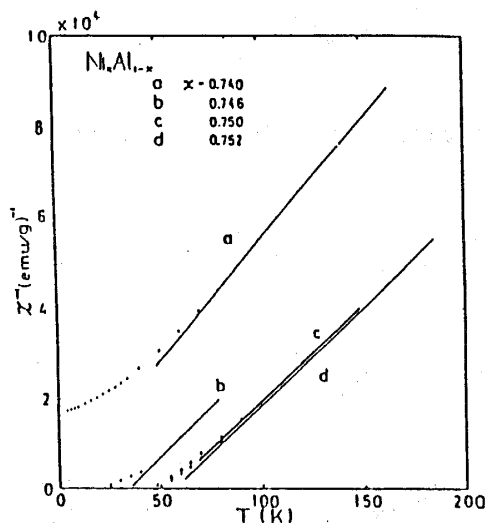
\text{Ni}_3\text{Al} 系における \chi^{-1} の温度依存性。
