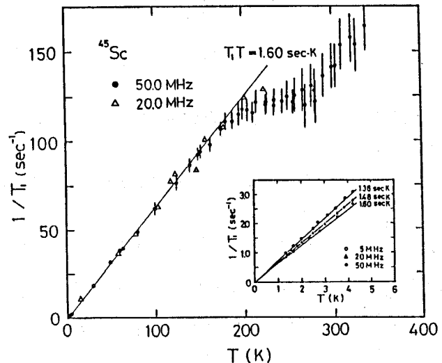
図 24 Sc 金属における ^{45}\text{Sc} の T_1^{-1} の温度依存性。実線は (T_1 T)^{-1} = 160 \text{ sec}^{-1} \text{ K}^{-1} 。1.3 と 4.2 K の温度範囲における T_1^{-1} の外部磁場依存性を挿入図に示す。
