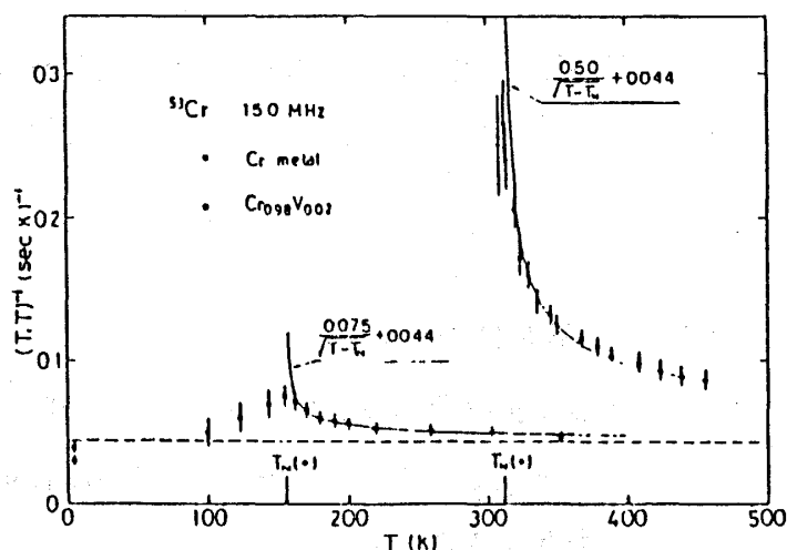
Cr金属と Cr_{0.98}V_{0.02} 合金の (T_1 T)^{-1} の温度依存性。破線は ^{53}Cr のコリン緩和率 (T_{1k} T)^{-1} の予測値を示す。
