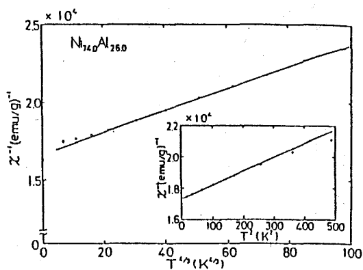
\chi^{-1} : T^{4/3} , \chi^{-1} : T^2 温度依存性。 \text{Ni}_{74.0}\text{Al}_{26.0} 合金について示す。
