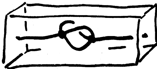
図3 「はめ込まれた三葉結び目」
