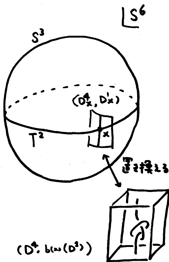
図4 Haefliger 結び目の生成元
