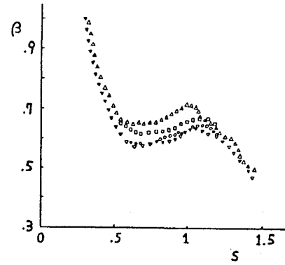
Fig. 4 1次相転移点近傍での内部エネルギーの振舞。 \triangle \cdots \beta_2/\beta_1=1, C_0=20, \Delta T=1000 \square \cdots \beta_2/\beta_1=1, C_0=10, \Delta T=2000 \cdots \beta_2/\beta_1=1, C_0=-20, \Delta T=1000 \circ \cdots \beta_2/\beta_1=1, C_0=-10, \Delta T=2000
