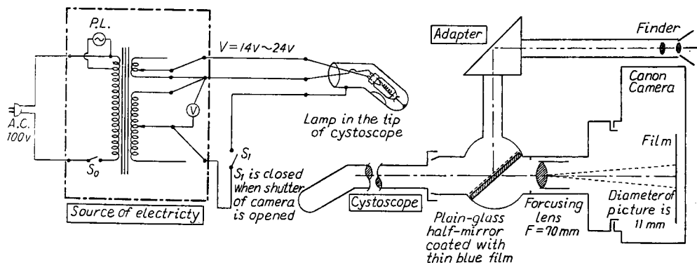
Fig. 1. Original apparatus.
