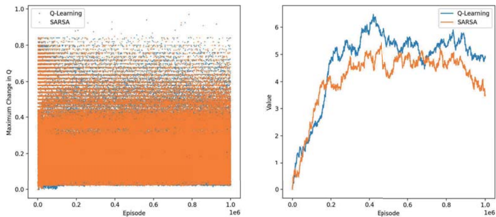
図 5 実装 B, Q-Learning ( \epsilon = 0.01 ), SARSA ( \epsilon = 0.01 ): 状態行動価値の最大更新量 (左), 状態 (1,0,0) の状態価値 (右)
