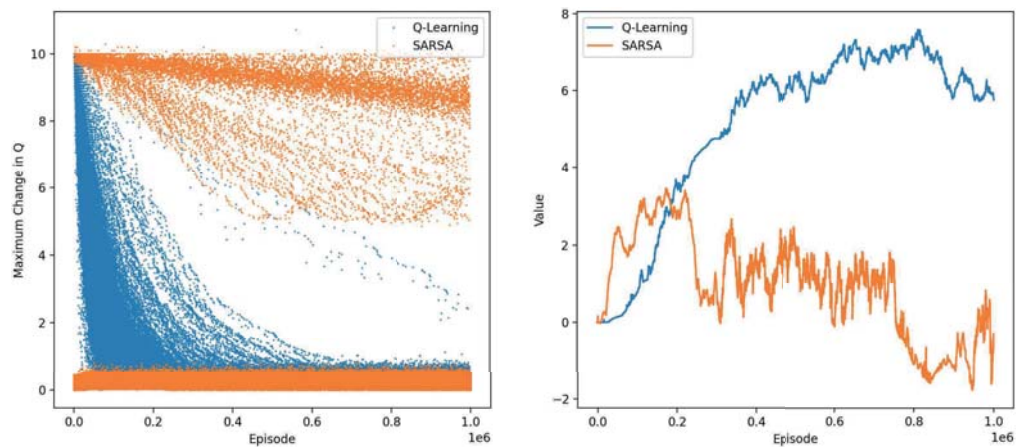
図 4 実装 A, Q-Learning ( \epsilon = 1 ), SARSA ( \epsilon = 0.01 ): 状態行動価値の最大更新量 (左), 状態 (1,0,0) の状態価値 (右)
