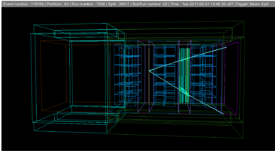
(b) CC1\pi^+ .
