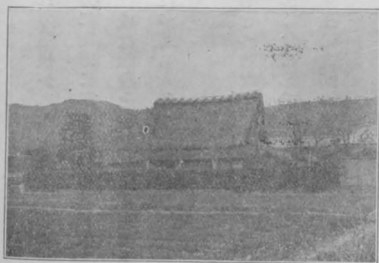
片入母屋茅葺 北嵯峨三宅忠一氏宅
