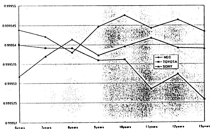
図 3.6 月次収益率の標本数変化に対する情報次元のに変化
