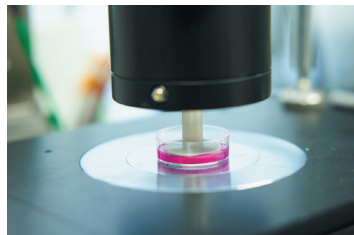
細胞を培養しているディッシュ内に音波を照射する装置
