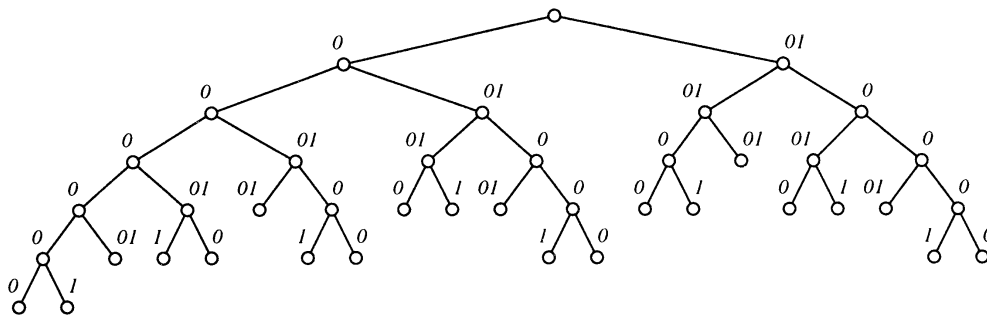
図 2 再帰木 \mathcal{F}_6
