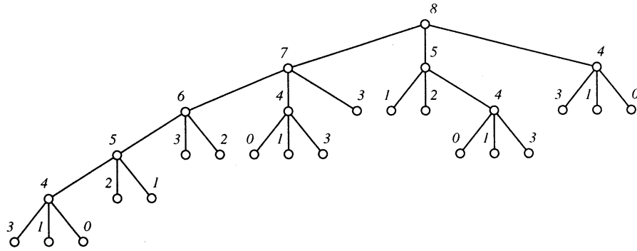
図 5 再帰木 \mathcal{P}_8
