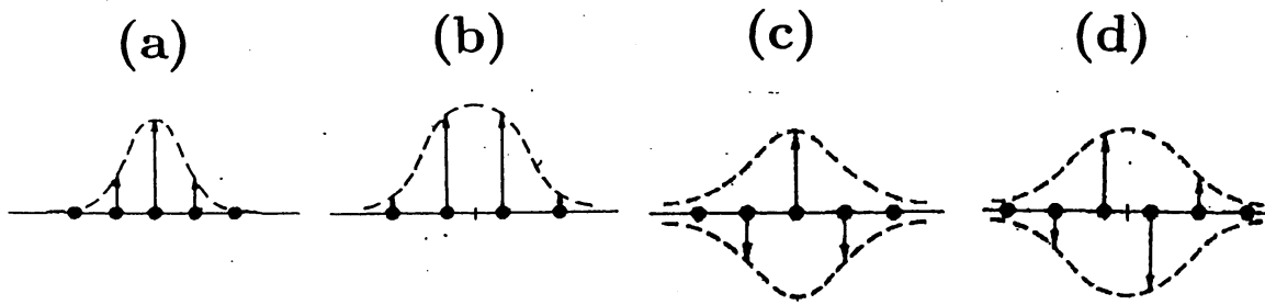
図4： 離散非線形シュレディンガー方程式の局在解 (a)(b) 低周波数モード (c)(d) 高周波数モード [(c),(d)は Sievers-Takeno モードと Page モードに対応]
