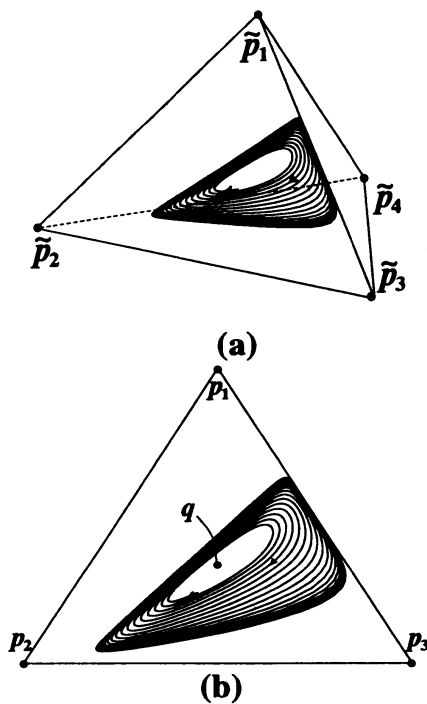
図 6: 新しく出現した周期軌道に漸近する軌道. 初期値は (\frac{5}{20}, \frac{6}{20}, \frac{6}{20}, \frac{3}{20}) . (a) は単体 S_3 上での軌道. (b) は軌道を S_y によって単体 S_2 へ射影した軌道.
