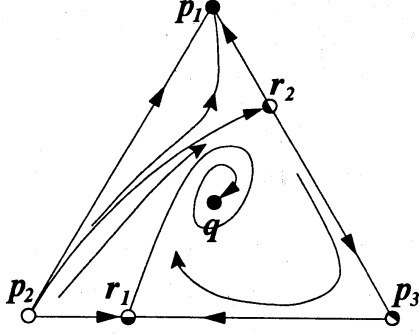
図 1: 単体 S_2 上のフローの構造. 2つの安定平衡点 p_1, q が存在し, それらの吸引領域の境界は p_2 から r_2 へのヘテロクリニック軌道となる.
