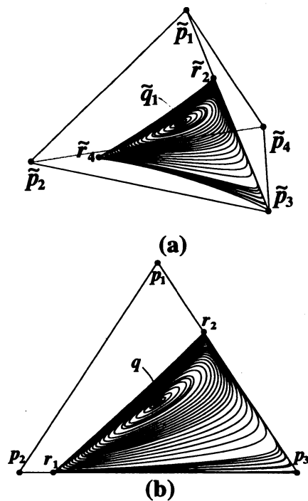
図 7: 不可算無限個の周期軌道からなるアトラクティングセット. (b) ではそれらを S_y によって元の相空間に射影している.
