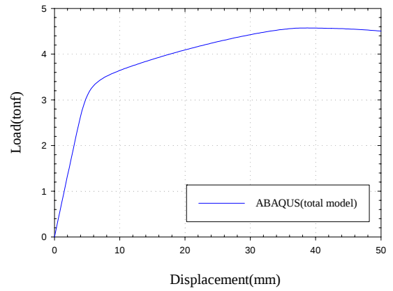
Fig. 5.30 Load-displacement (Case-4)
