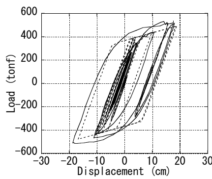
(b) Load-displacement
