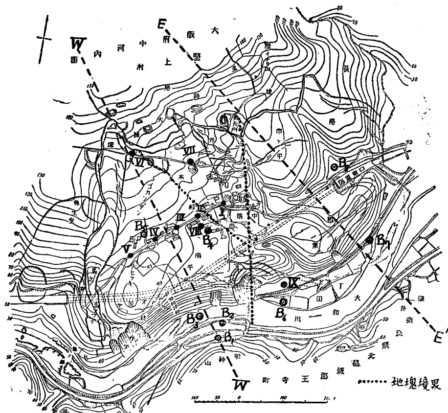
第1圖 堅上村特區の地形と電氣抵抗測定地點 (I~IX) 並に内務省のボーリング地點 ( B_1 \sim B_8 )
