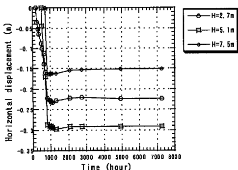
Fig. 4 Horizontal displacement
