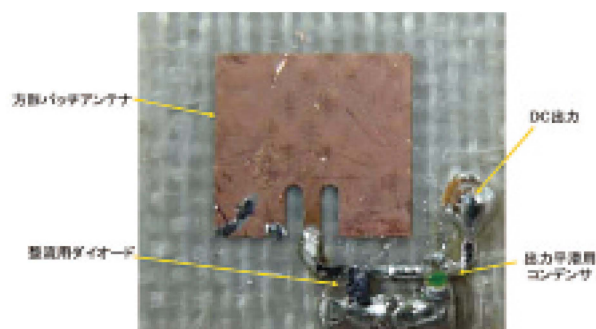
開発された24GHzレクテナ(2009)
