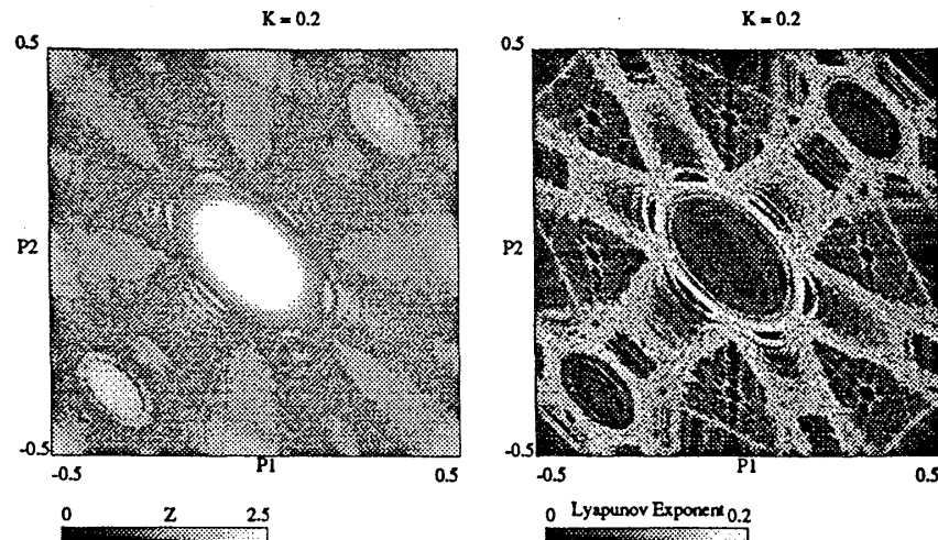
(a) クラスター状態の分布 (白い部分がクラスターになる初期状態)
