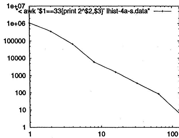
Figure 3: 2 binars 状態の寿命分布 (両対数)。横軸は寿命 / 512, 縦軸は頻度。およそ 1/\tau^2 のべき分布
