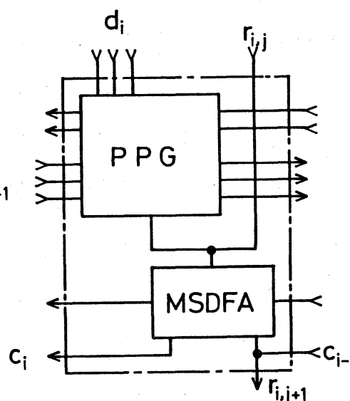
図 7 除算モジュール
