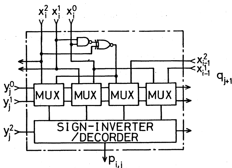
図 6 部分積生成回路 (PPG)
