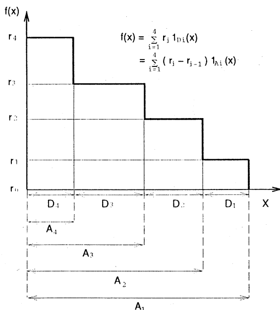
図 2.4: 単関数 f
