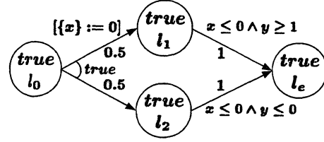
図 1: 確率時間オートマトン G_1
