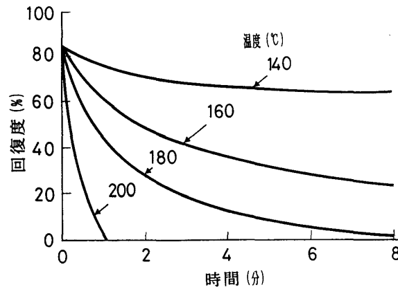
図10 圧縮度51%のスギ圧縮材を水蒸気処理したものの回復度と水蒸気処理時間の関係 18)
