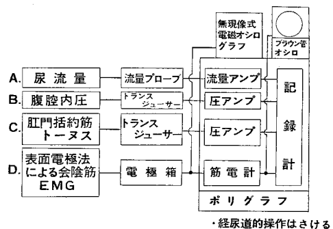
Fig. 2. 非経尿道的、非経膀胱的手技による尿水力学的検査法
